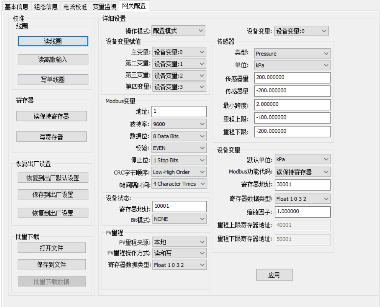
图 2.4 网关配置选项卡
