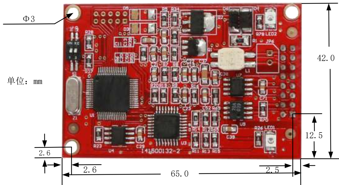
图 1.4 HART 模块正面机械尺寸图
