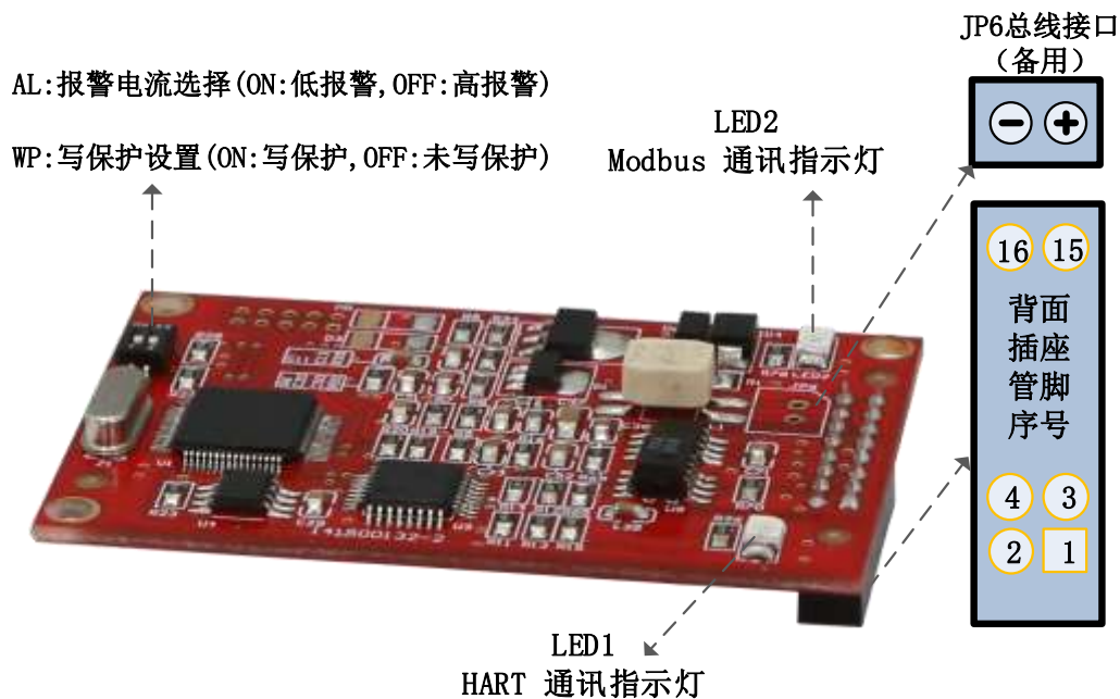
图 1.3 硬件用户接口示意图
